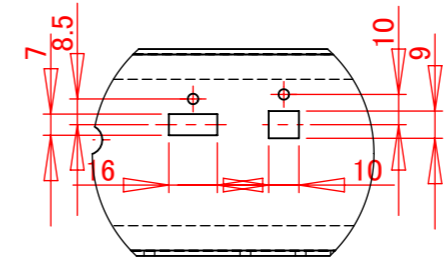
詳細図 A スケール 2 : 5
